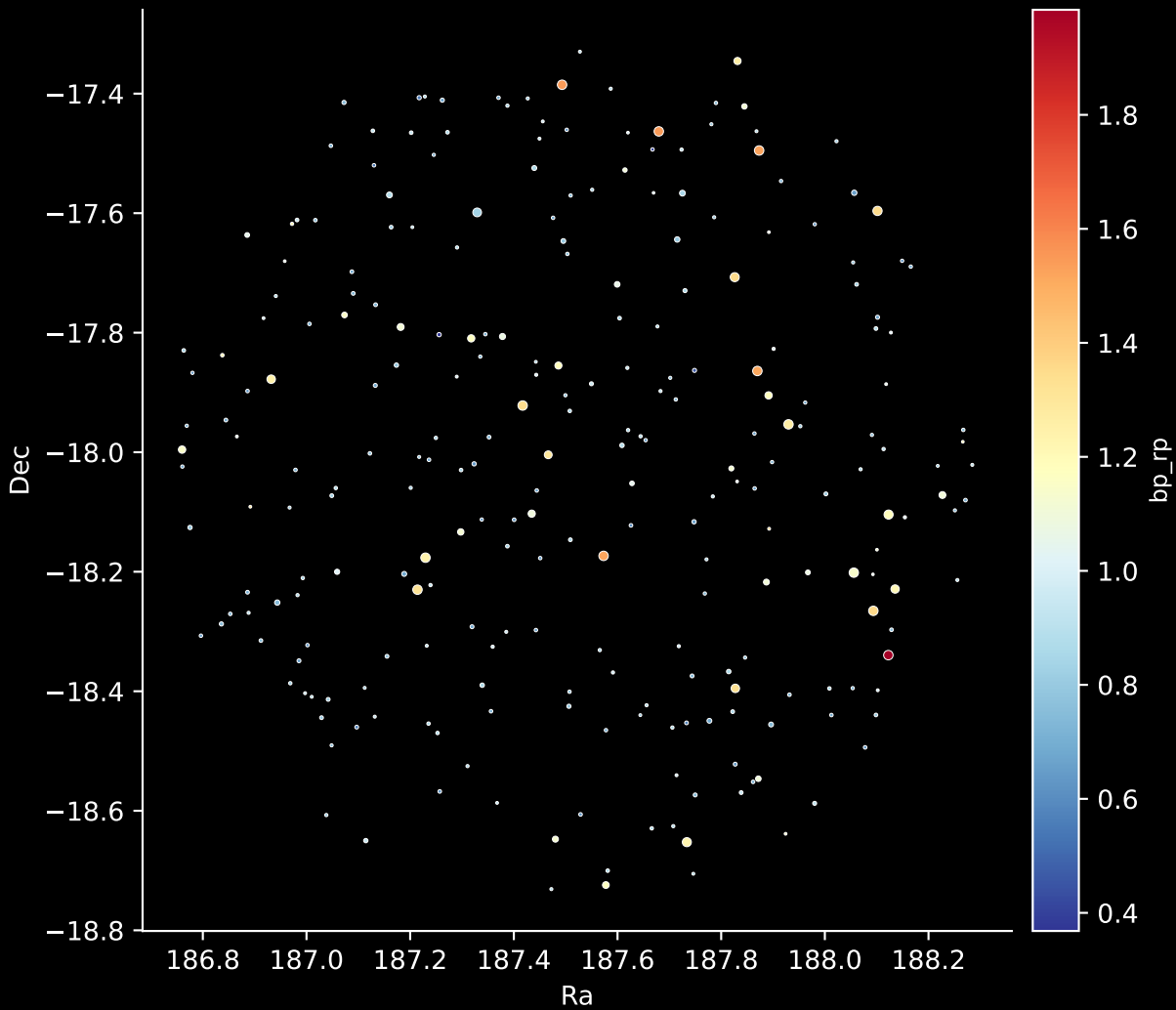
GALAH DR4 Field: [1948] Stars: 257
