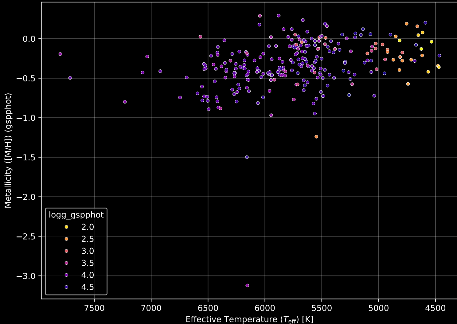
GALAH DR4 Field: [1948] Stellar Population Parameters (n= 257)
