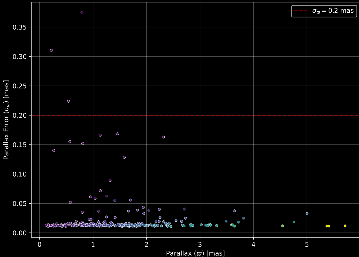
GALAH DR4 Field: [1948] Parallax Quality (n= 257)
