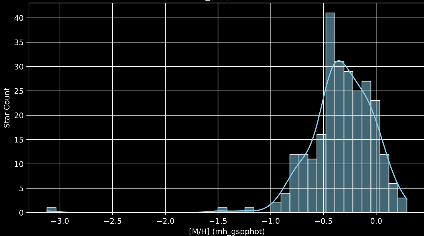
GALAH DR4 Field: [1948] [M/H] (mh_gspphot) (n= 257)
