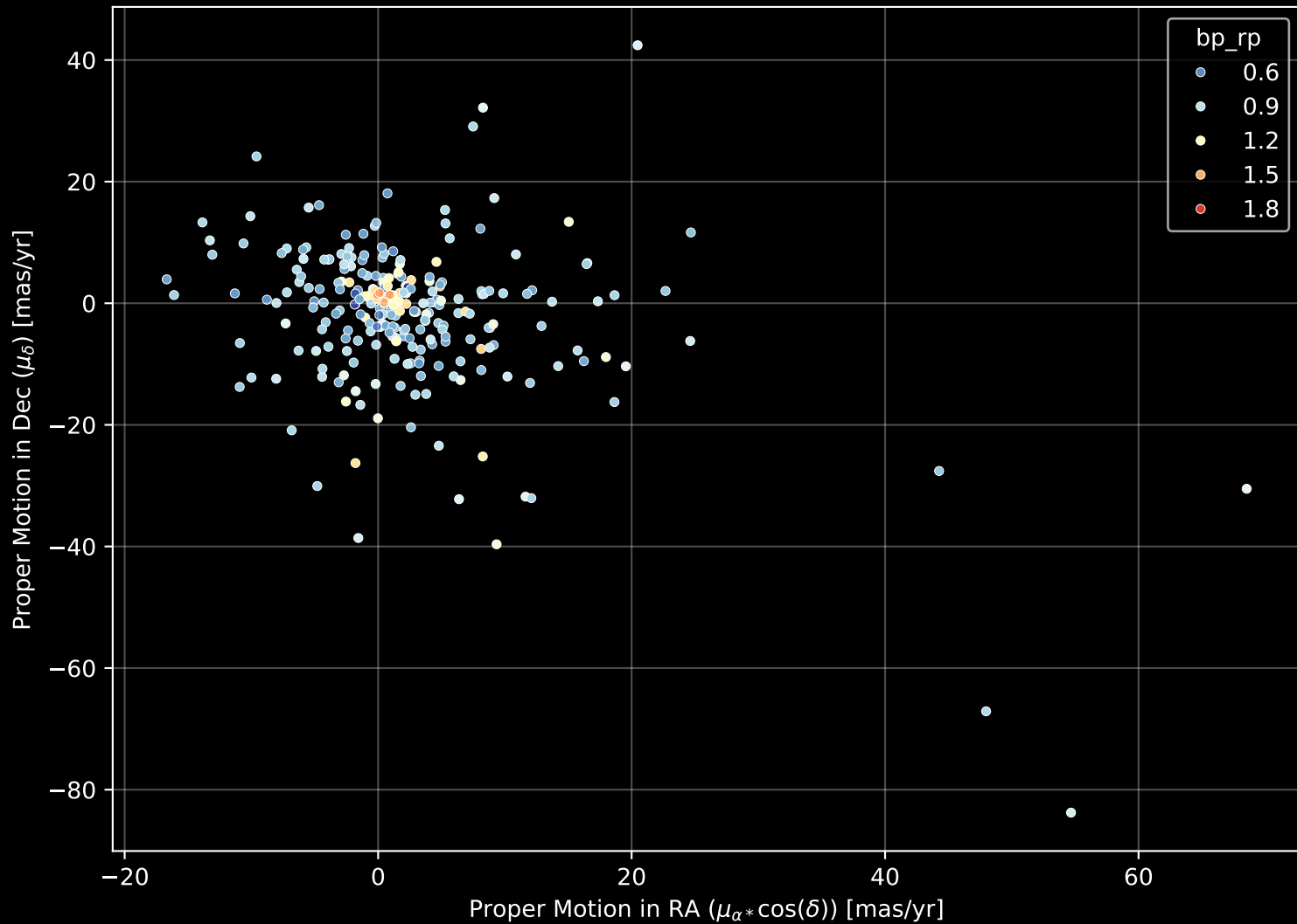
GALAH DR4 Field: [1948] Proper Motion Diagram (n= 257)
